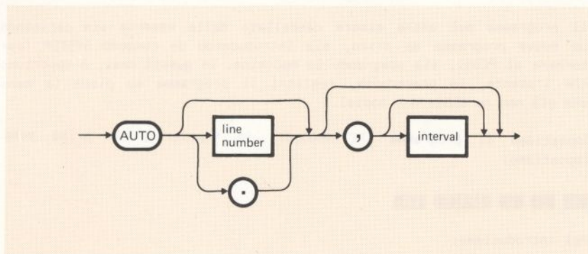
Figura 2-3 Comando AUTO
